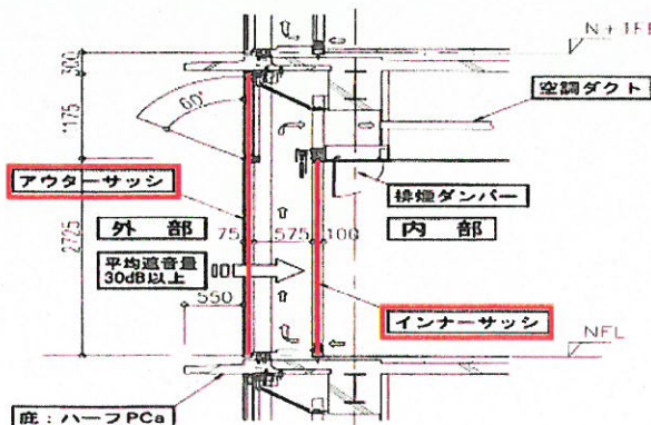
(図-1) ダブルスキン断面図
