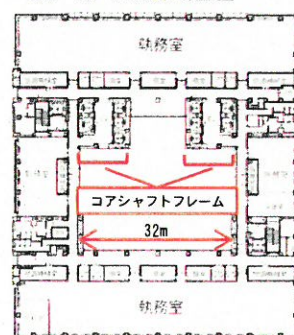
（図-2）基準階平面図
