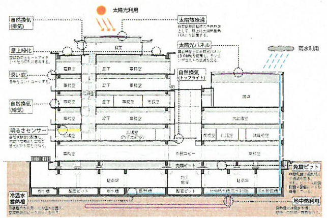
■断面図：工口技術説明図
