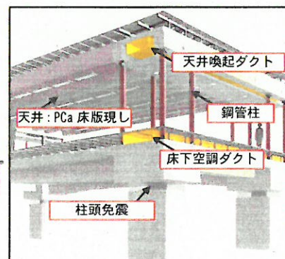
(図-2) 構造基本構成
