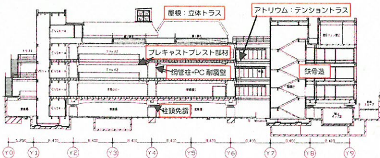
(図-1) 断面図
