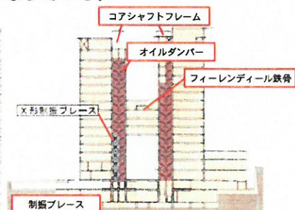
（図-1）行政棟断面図
