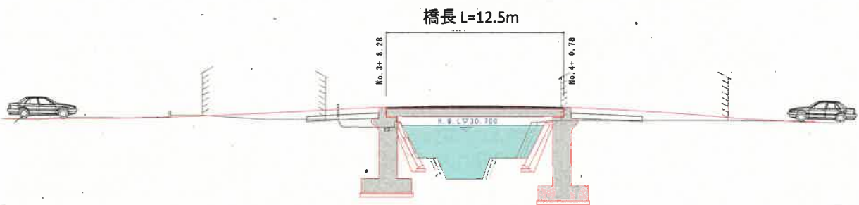
縦断面図
