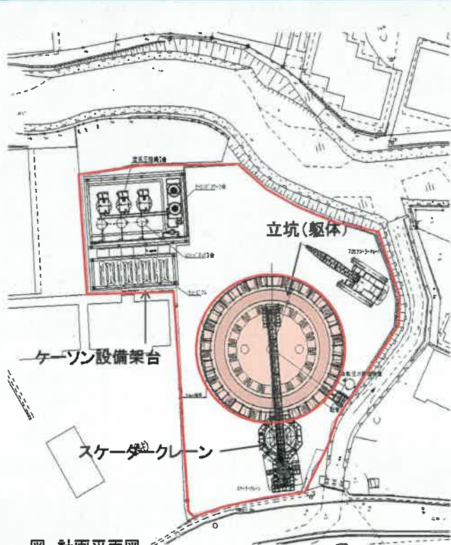
図 計画平面図
