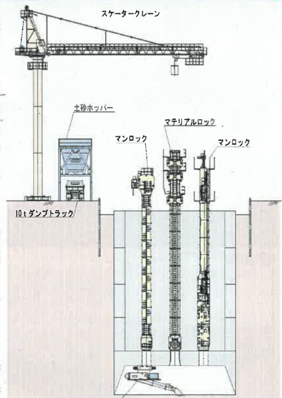
図 ニューマチックケーソンイメージ図
